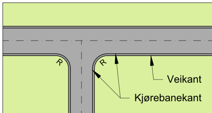
Figur 5.28: Tilslutningsradier mellom kjørebane kantene i et veikryss
