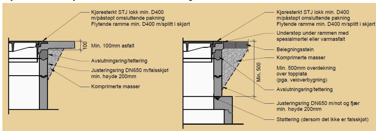
Figur 7.9: Detalj for asfaltering ved kumlukk i flyteramme
